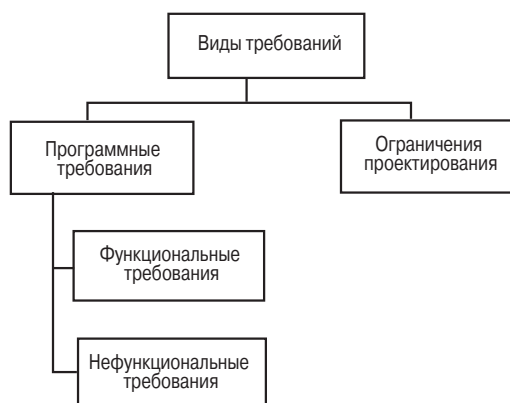
Рис. 23.3. Типы требований
