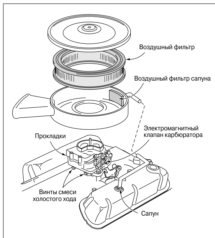
Рис. 3.1. Воздушный фильтр находится внутри воздухоочистителя
