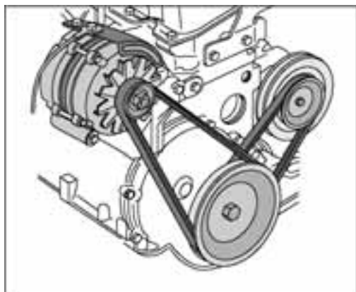
Рис. 3.2. Ремни
